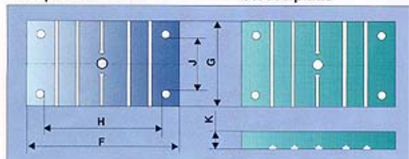
Stößelplatte
